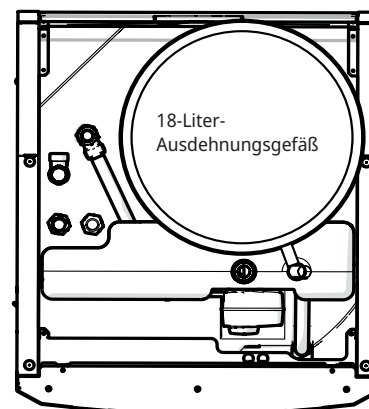
Draufsicht
