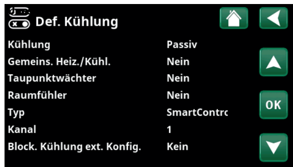
Menü: „Fachmann/Definieren/Kühlung“.
