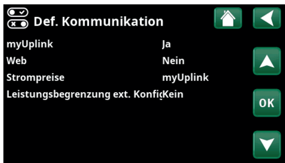
Menü: „Fachmann/Definieren/Kommunikation“.
