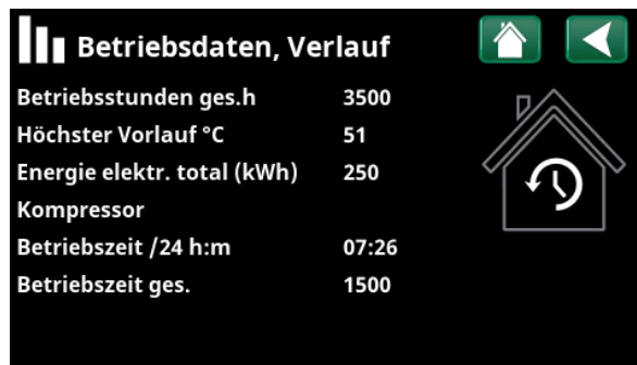
Menü: „Betriebsdaten/Verlauf“.
