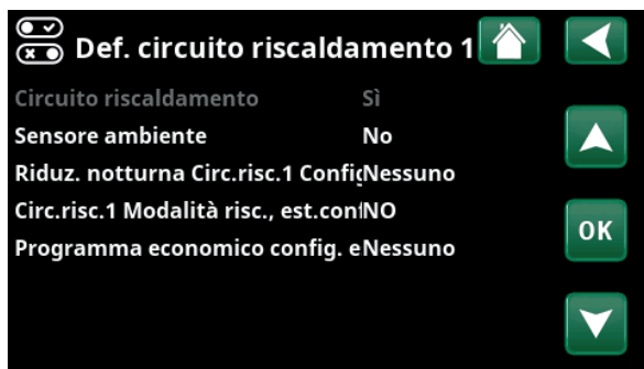
Menu "Avanzato/Definire/Circuito riscaldamento/Circuito riscaldamento 1".
